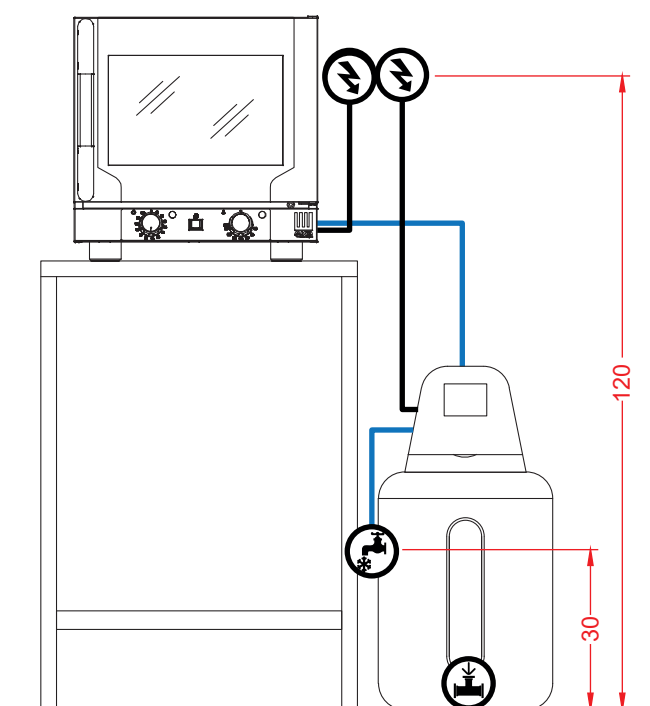
Vista Elevación
