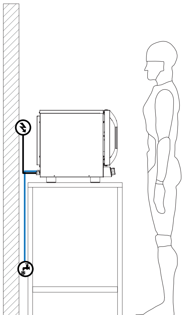
Vista Izquierda
