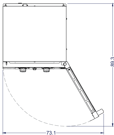
Vista Planta
